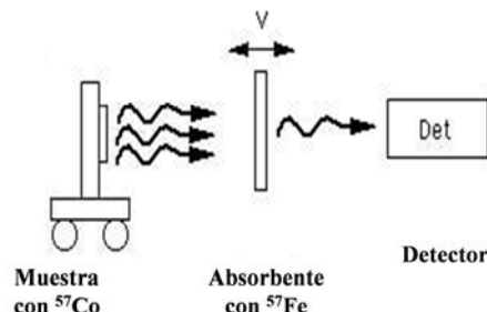
Figura 2: Geometría del arreglo de la Espectroscopía Mössbauer en el Modo de Emisión.
