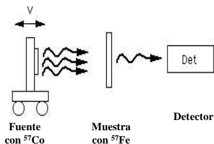
Figura 1: Geometría del arreglo de la Espectroscopía Mössbauer en el Modo de Transmisión
