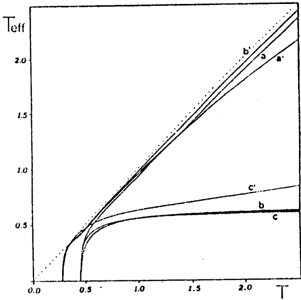
Figura 1b: (a), (b), y (c) denotan las temperaturas efectivas asociadas a los operadores J_z , Q , Q y (J_z^2 + J_x^2)/2 respectivamente en el tratamiento de HFG estadístico, mientras que (a'), (b') y (c') denotan las mismas cantidades en la aproximación de orden superior.
