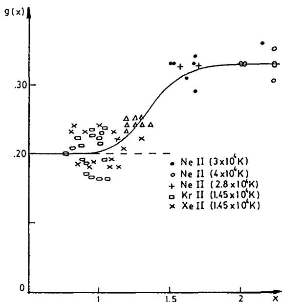
Figura 1: Valores experimentales del factor de Gaunt para transiciones ns-np de la tabla 1 y de referencias 2 y 6. La curva continua está dada por la ecuación (6).
