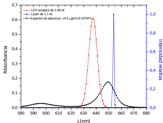
Figura 3. Solapamiento entre Láser de Diodo de 1,1 W y LED de 1,06 W contra la curva de absorción de la mTHPC
