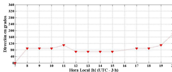
Figura 7: Dirección del viento para la ciudad de Comodoro Rivadavia el 21 de enero de 2015- AR_ASOS Network.
