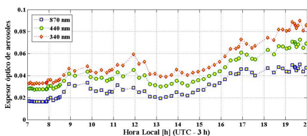
Figura 8: Evolución temporal del espesor óptico de aerosoles para la ciudad de Comodoro Rivadavia el día 21 de enero de 2015.
