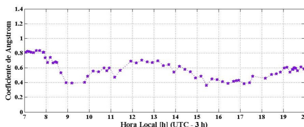
Figura 9: Evolución temporal del Coeficiente de Ångström para la ciudad de Comodoro Rivadavia el día 21 de enero de 2015.
