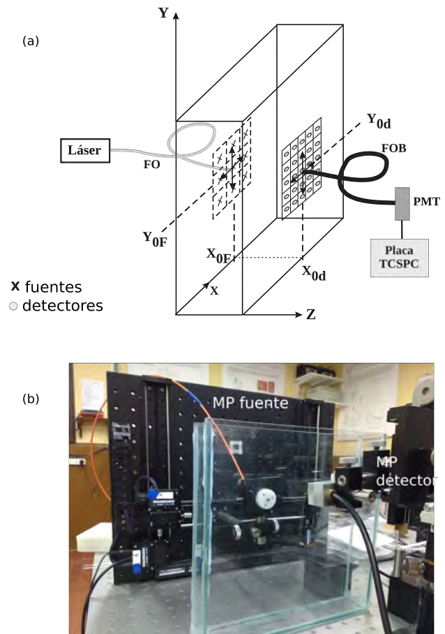
FIG. 1: Esquema del arreglo experimental de las medidas tipo tomográficas.
