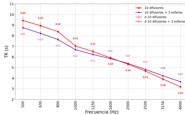
FIG. 7: tiempos de reverberación de la cámara sin la muestra ( TR_1 ). Cada punto es resultado de un promedio sobre 12 posiciones para el par micrófono/altavoz, con su correspondiente incertidumbre.
