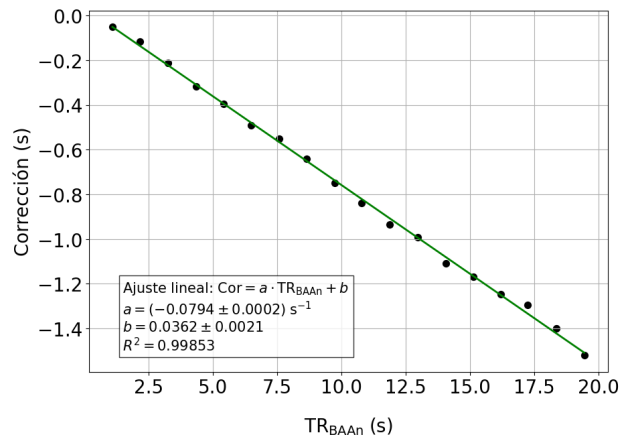
FIG. 8: corrección en función del tiempo de reverberación medido con el BAA. En verde, ajuste lineal por cuadrados mínimos ponderados.
