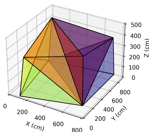
FIG. 2: tetraedralización de Delaunay, se muestran los 7 tetraedros en colores distintos.
