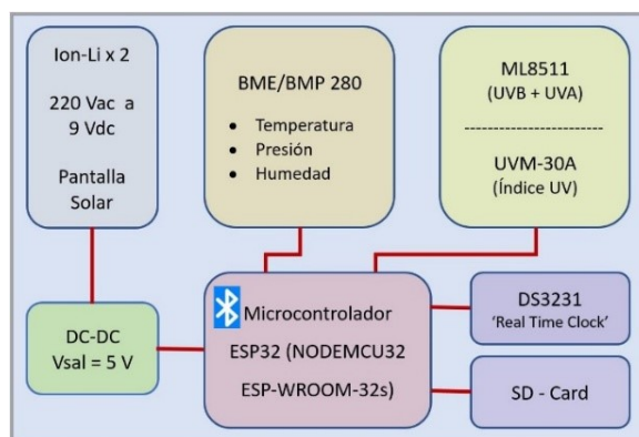
FIG. 1: Diagrama esquemático del Prototipo Implementado
