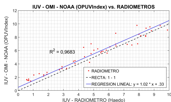
FIG. 11: Calibración entre los datos provistos por el OMI-NOAA y los datos adquiridos con el Radiómetro de Haedo (corresponden a las mismas fechas y horas del 2024)
