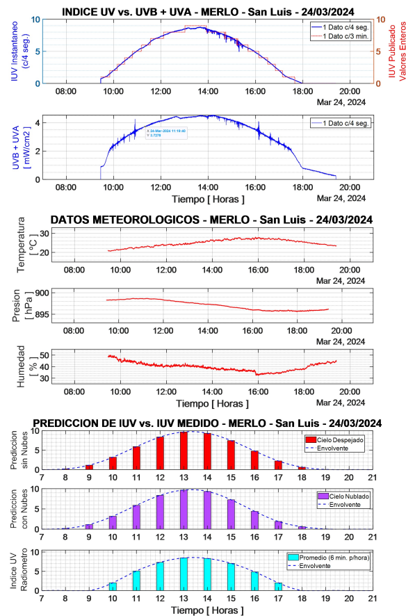
FIG. 7: Resultados obtenidos el 24/03/2024 en Carpintería – San Luis a 1350 metros de altitud con los datos meteorológicos locales y la predicción del SMN – Cielo despejado.
