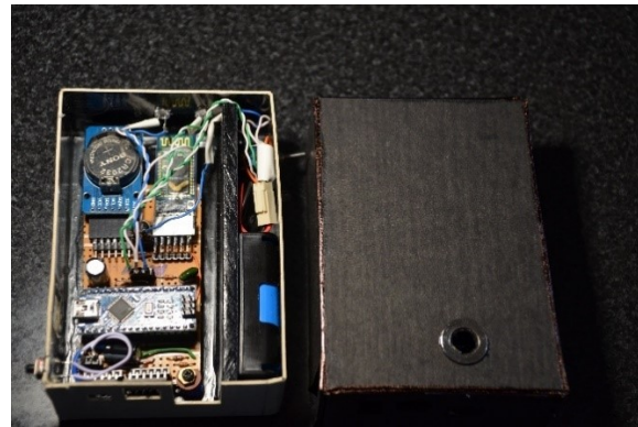
FIG. 3: Prototipo funcional de unidad portátil
