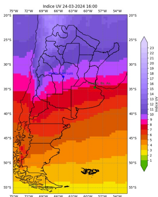
FIG. 8: Mapa del IUV en la Argentina para el 24/03/2024 al mediodía solar (13:00 hora oficial. – 16:00 UTC).
