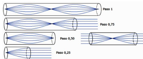
Figura 3. Esquemas de medios GRIN con diferentes pasos.
