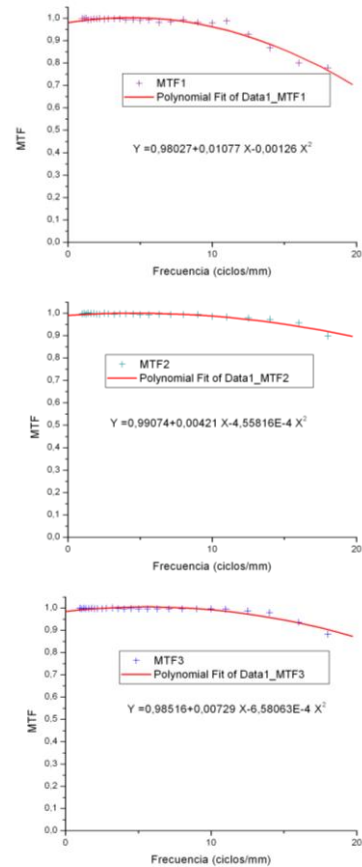
Figura 9. Resolución de los tres medios GRIN para las frecuencias contenidas en la Edmund Optics NBS 1963 utilizada
